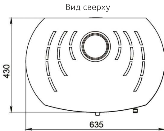
Рис. 6. Габаритные размеры печи-камина «СИБИРЬ-10»
